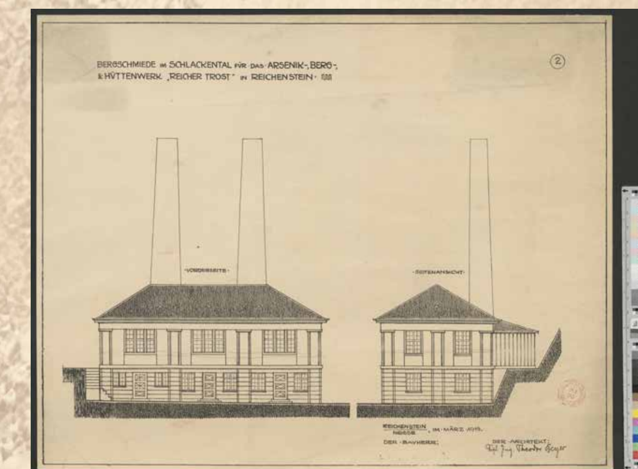
SZKIC ZABUDOWAŃ KUZNI ZAKŁADÓW ARSENOWYCH W ZŁOTYM STOKU. PROJEKT THEODORA BEYERA, ROK 1919 ARCHIWUM PAŃSTWOWE WE WROCŁAWIU, ZESPÓŁ 82/244/O WYŻSZY URZĄD GÓRNICZY WE WROCŁAWIU (OBB BRESLAU), SYGN. II/152
