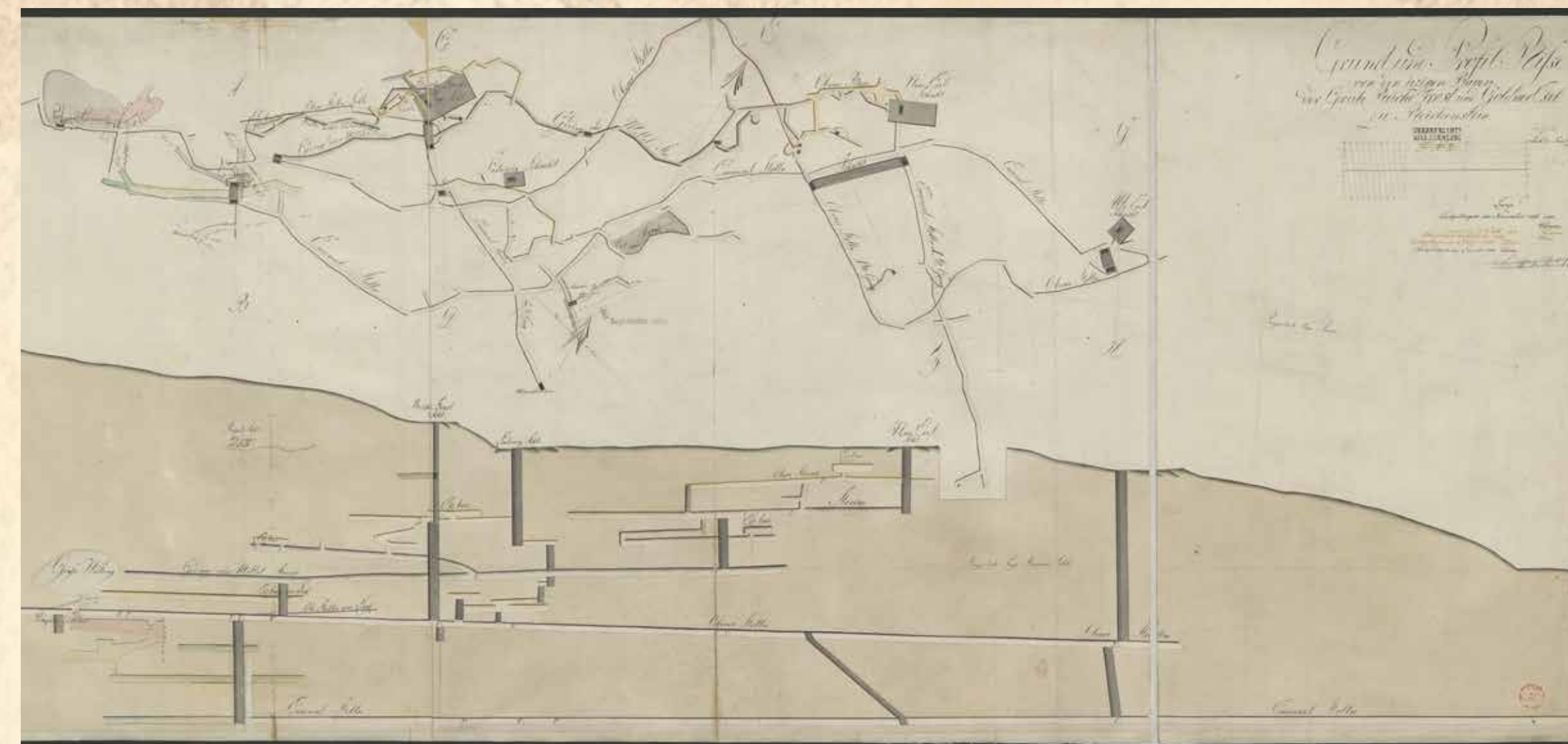
MAPA POKŁADÓW PÓLA „BOGATE POCIESZENIE” (REICHE TROST) ORAZ „ZŁOTY OSIÓŁ” (GRUND UND PROFIL REISE DER GRUBE REICHE TROST UND GOLDNER OSEL ZU REICHENSTEIN), 1806-1811 ARCHIWUM PAŃSTWOWE WE WROCŁAWIU, ZESPÓŁ 82/244/O WYŻSZY URZĄD GÓRNICZY WE WROCŁAWIU (OBB BRESLAU), SYGN. II/120
