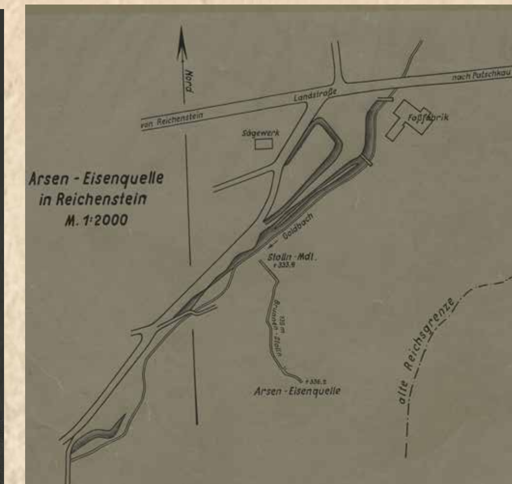
SZKIC SYTUACYJNY SZTOLNI ARSENOWEJ (OCHROWEJ), OKRES MIĘDZYWOJENNY ARCHIWUM PAŃSTWOWE WE WROCŁAWIU, ZESPÓŁ 82/244/O WYŻSZY URZĄD GÓRNICZY WE WROCŁAWIU (OBER BERGAMT BRESLAU), SYGN. II/131
